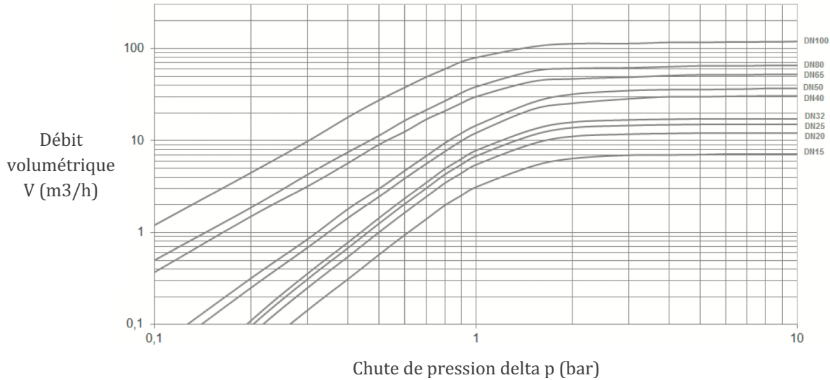
Diagramme de débit eau
