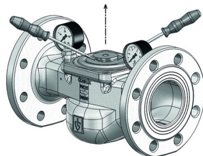
Figure B) : Retirer l'unité de régulation DN65-DN80
